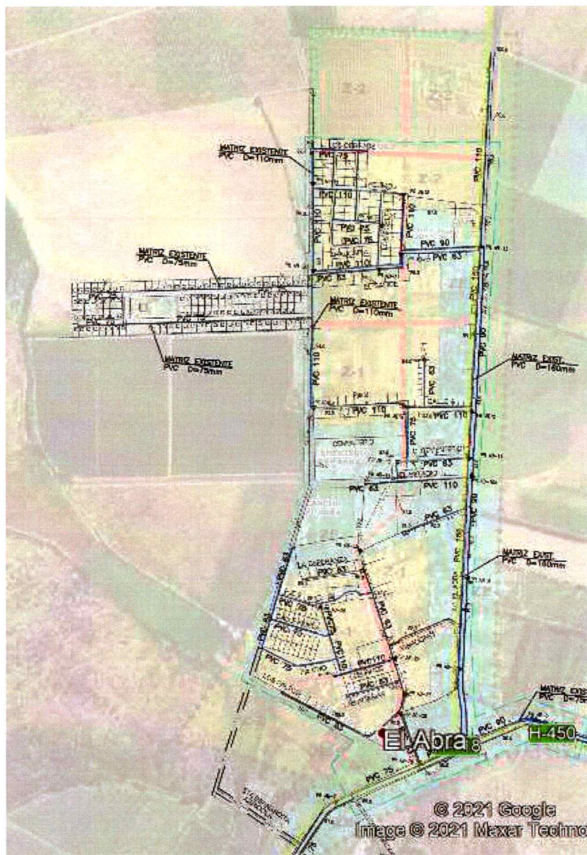
Imagen nº3.4 Distribución de Redes APR EL ABRA. FUENTE: ELABORACION PROPIA EN BASE A INFORMACION PROPORCIONADA POR EL APR.
