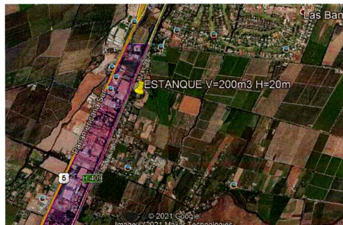
Imagen n°3.6 Ubicación de Sondaje N°1 y n°2 y Estanque. FUENTE: ELABORACION PROPIA EN BASE A INFORMACION PROPORCIONADA POR EL APR.
