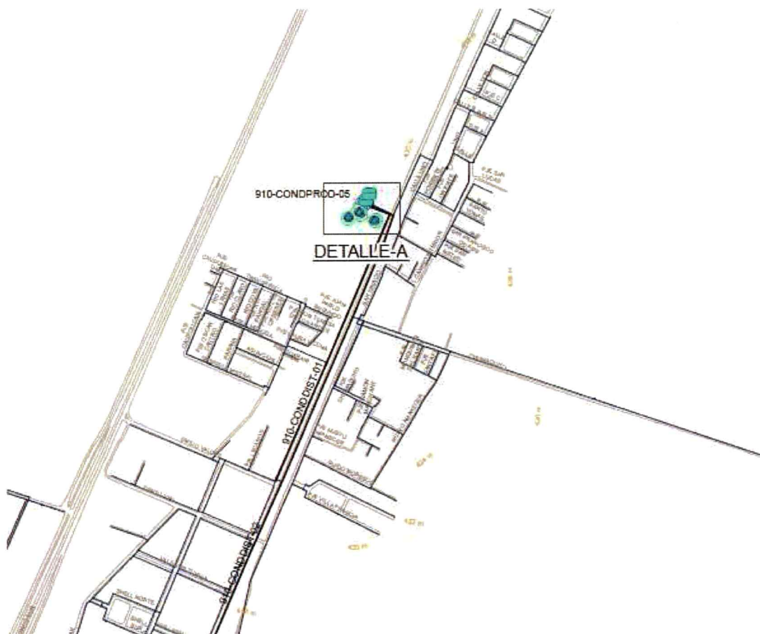
Imagen nº 2.1 Ubicación Sondajes. Fuente PD ESSBIO 2019.
