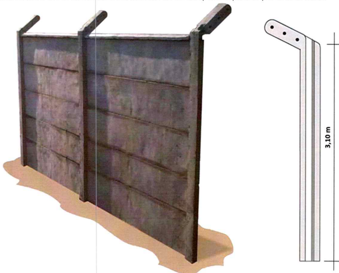
Imagen Referencial: Pandereta 5 placas / Pilar curvo (cabeza de caballo) h=3,1 m
