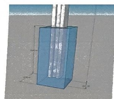
FUNDACION POSTE AISLADO
