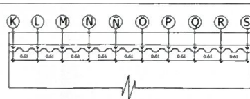
Elevación Posterior
