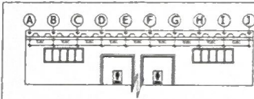
Elevación Principal
