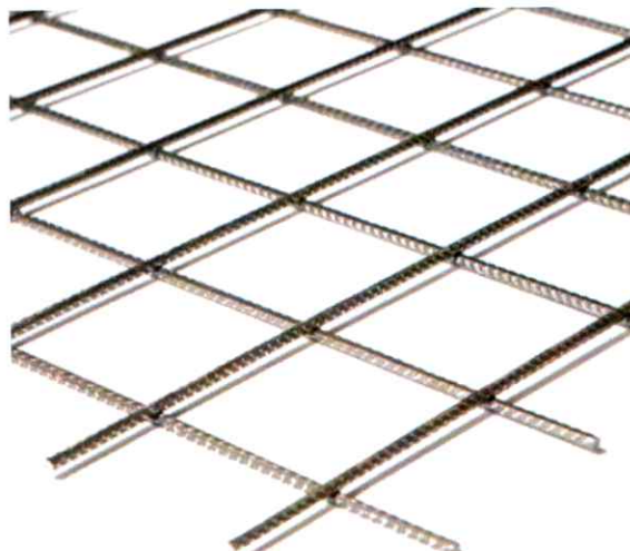
IMAGEN REFERENCIAL: Placa colaborante galvanizada de 0,8 x 950 mm x 6 m / Malla electro soldada C-92 de acero AT56-50H.
