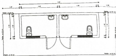
Planta Arquitectura
