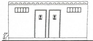
Elevación Principal
