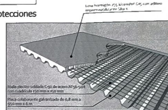
Losa Colaborante - Cubierta
