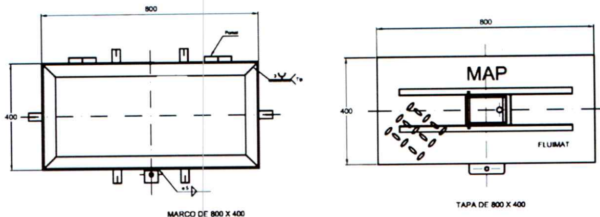
IMAGEN REFERENCIAL: TAPA GUARDAMEDIDOR 800 x 400 mm – ACERO DIAMANTADO GALVANIZADO.
