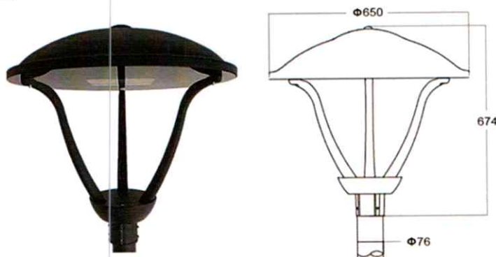
IMAGEN REFERENCIAL: LUMINARIA LED PAGODA ISLAND 60 W, LUZ FRÍA.
