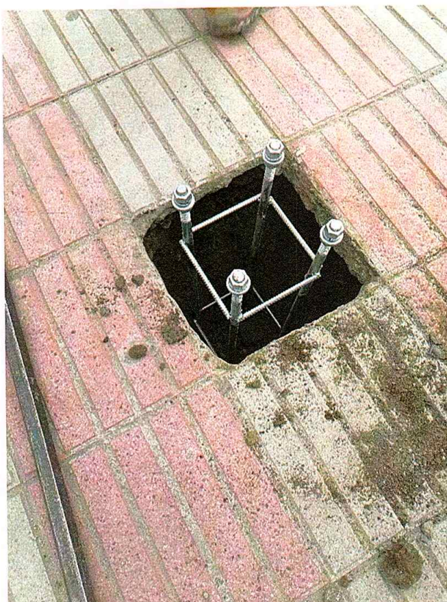
Ilustración 4 "Canastillo instalado en fundación"
