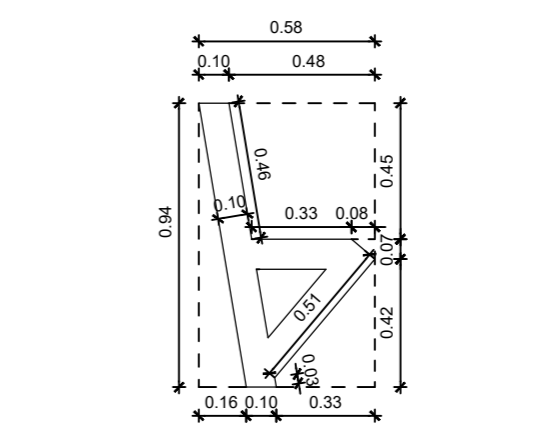
Trazado Banca Paradero Escala 1 : 25
