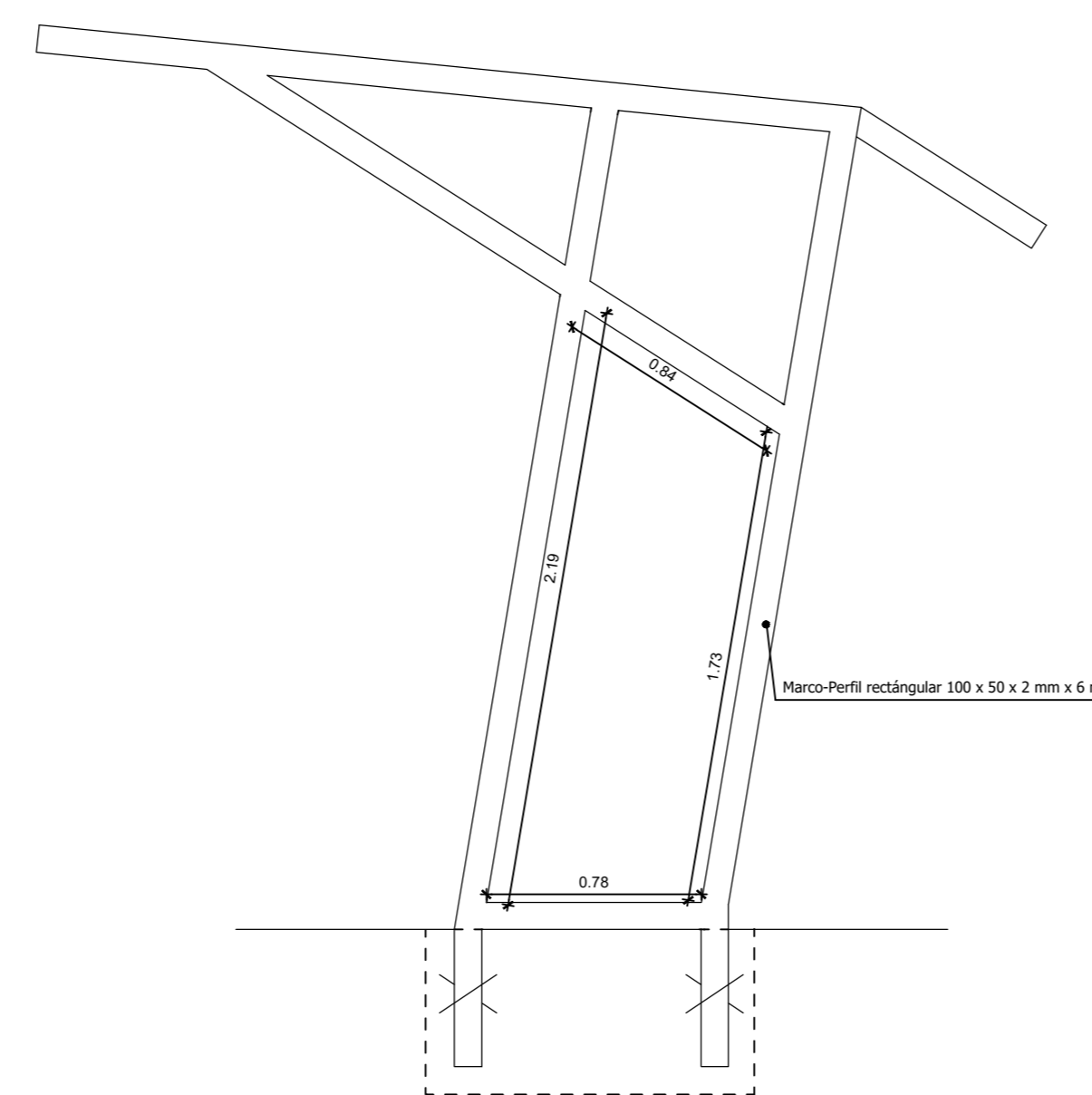
Elevacion Marco Paradero Escala 1 : 25
