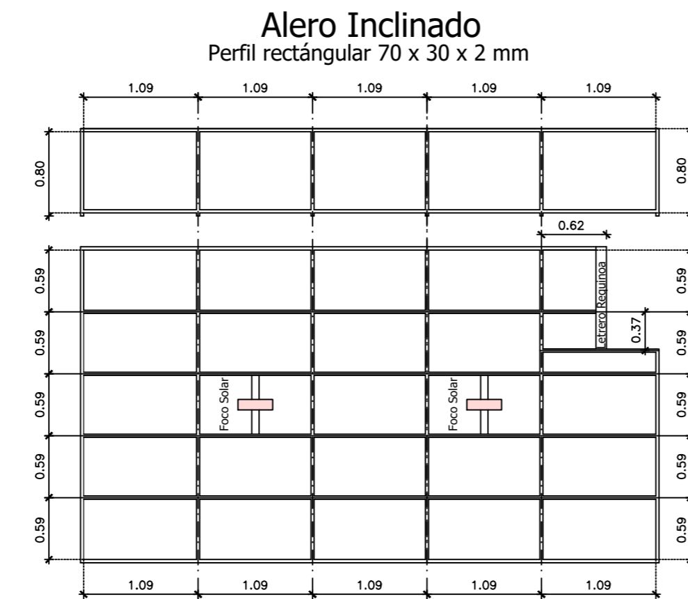
Planta de Techumbre Perfil rectangular 70 x 30 x 2 mm Escala 1 : 50
