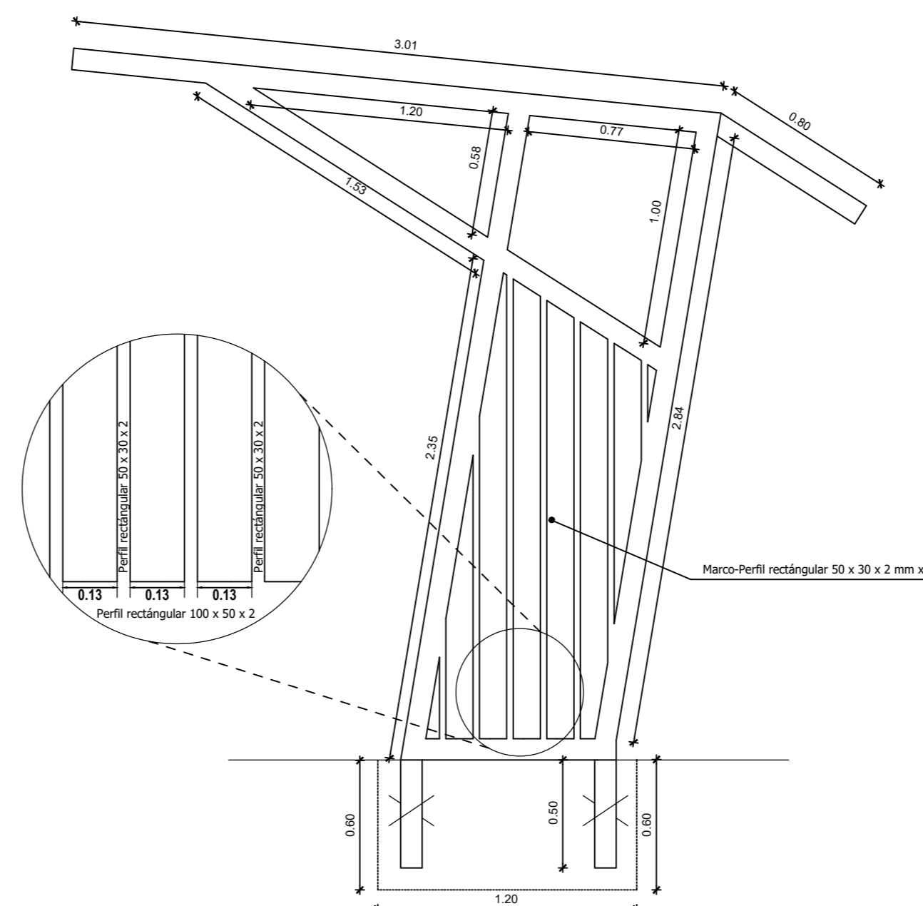
Detalle Marco Paradero Escala 1 : 25
