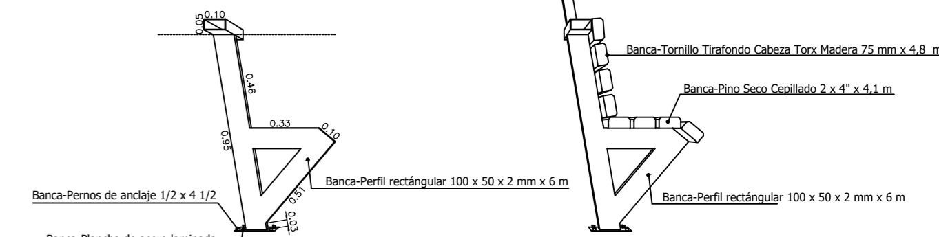
Elevacion Banca Escala 1 : 25
