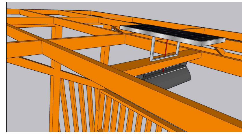
Detalle Panel y Foco Solar ESCALA 5:1
