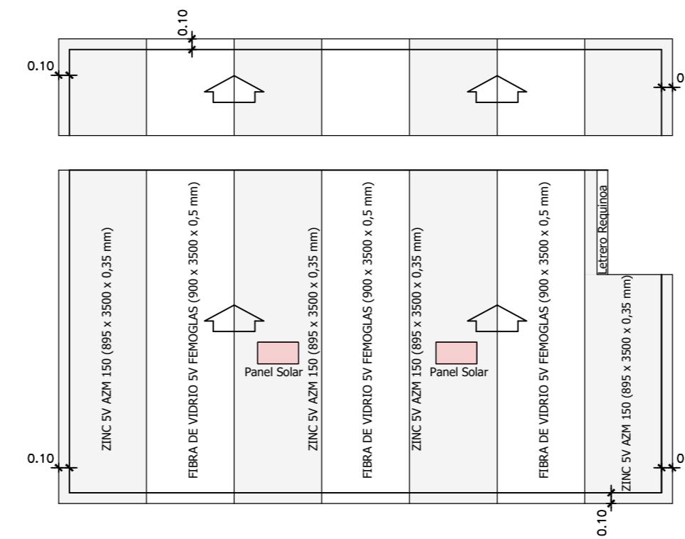
Planta de Cubierta Perfil rectangular 70 x 30 x 2 mm Escala 1 : 50
