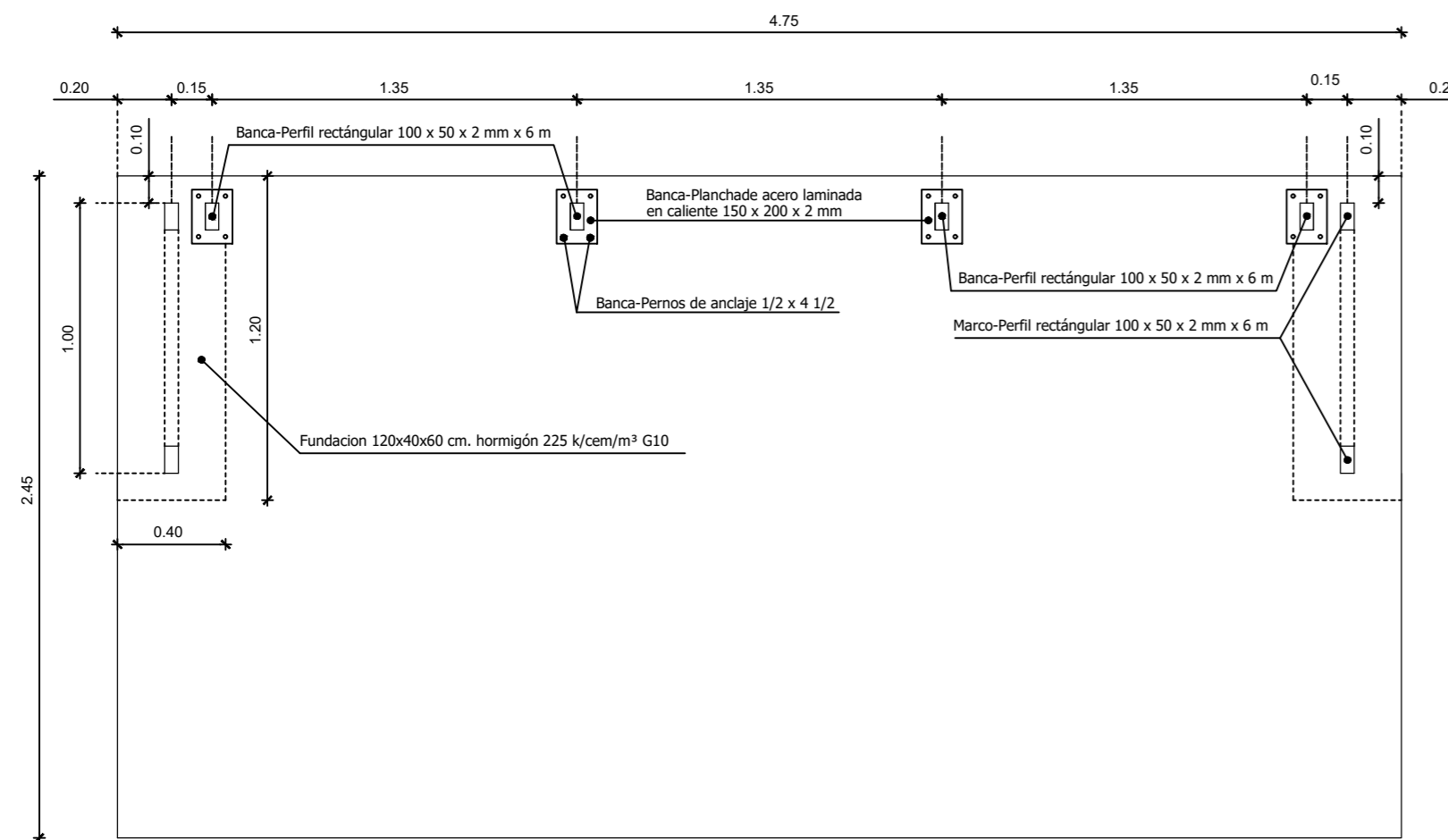
Planta Fundaciones y Estructuras Escala 1 : 25
