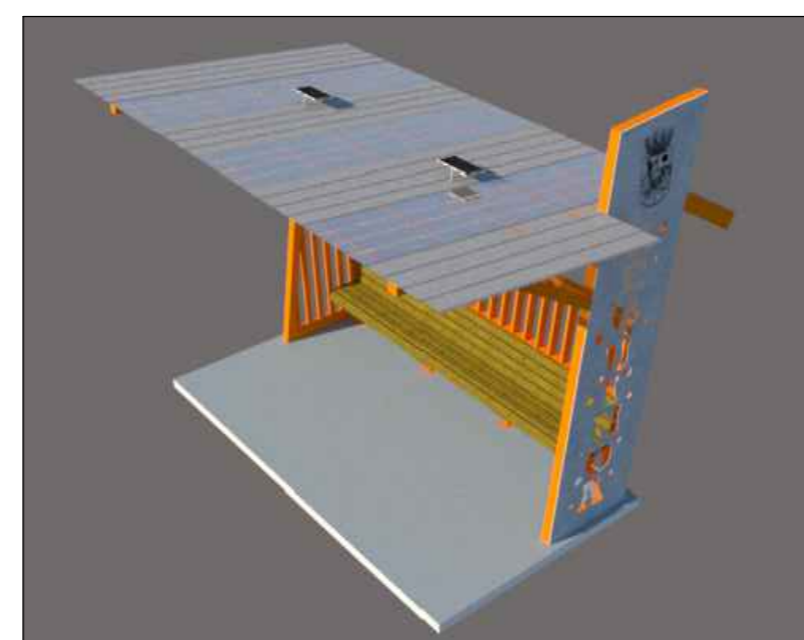
Vista Cubierta Paradero ESCALA 5:1
