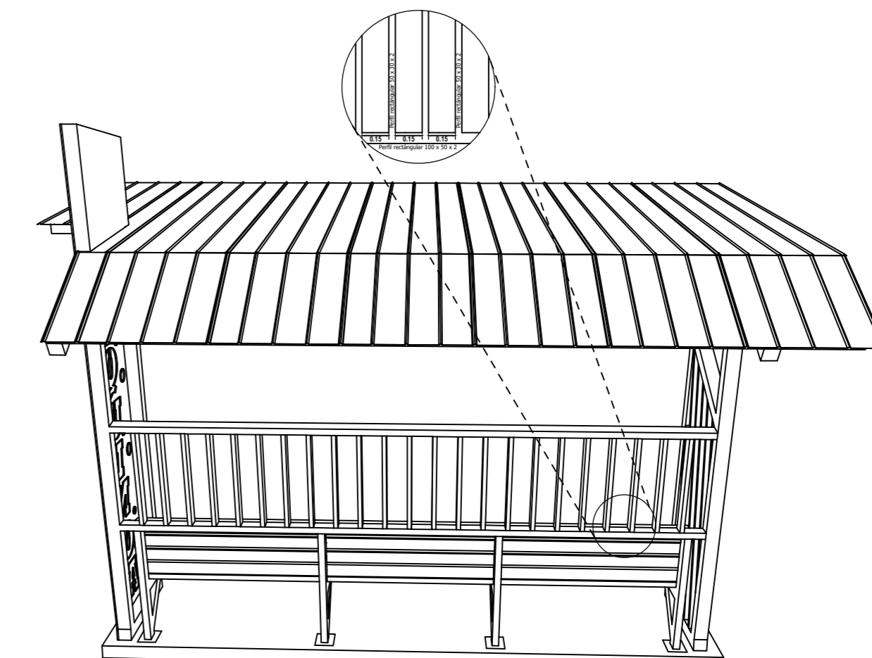
Elevacion Posterior Paradero Escala 1 : 25
