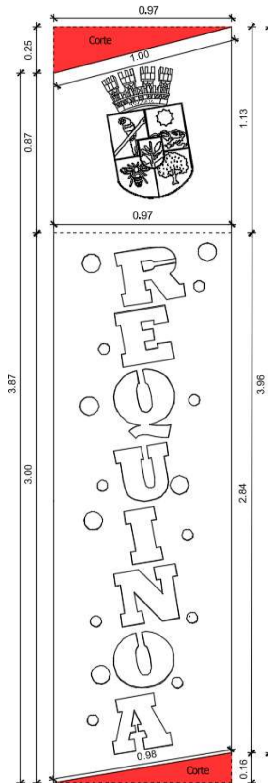
Modelo de letrero. Plancha acero inoxidable 6mm. Técnica de letras: corte laser. Técnica de escudo: grabado laser.
