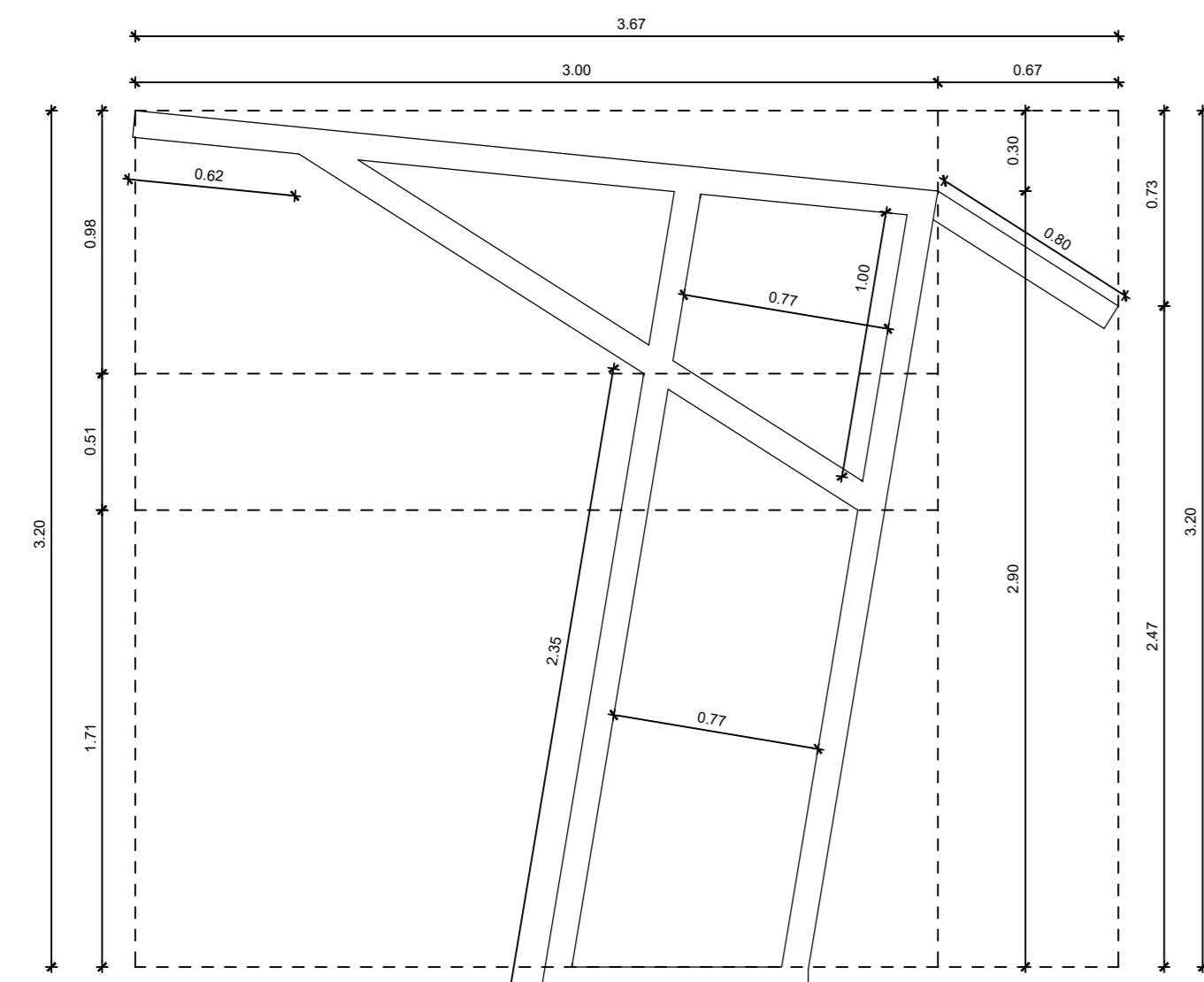
Planta Fundaciones y Estructuras Escala 1 : 25
