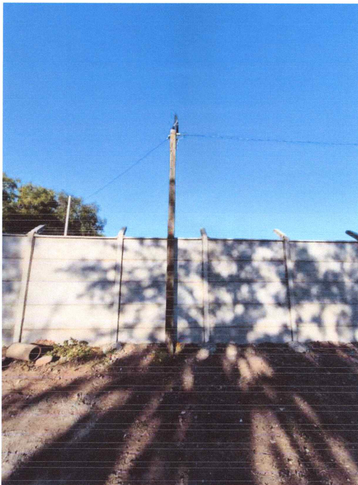
IMAGEN 36: SIN ITEM: REINTALACION DE POSTE PARA SOPORAR RED PUBLICA QUE ALIMENTA LUMINARIAS QUE APUNTAN HACIA SITIO ERIAZO ADYACENTE A LA PANDERETA TRASERA DE LOS BAÑOS.
